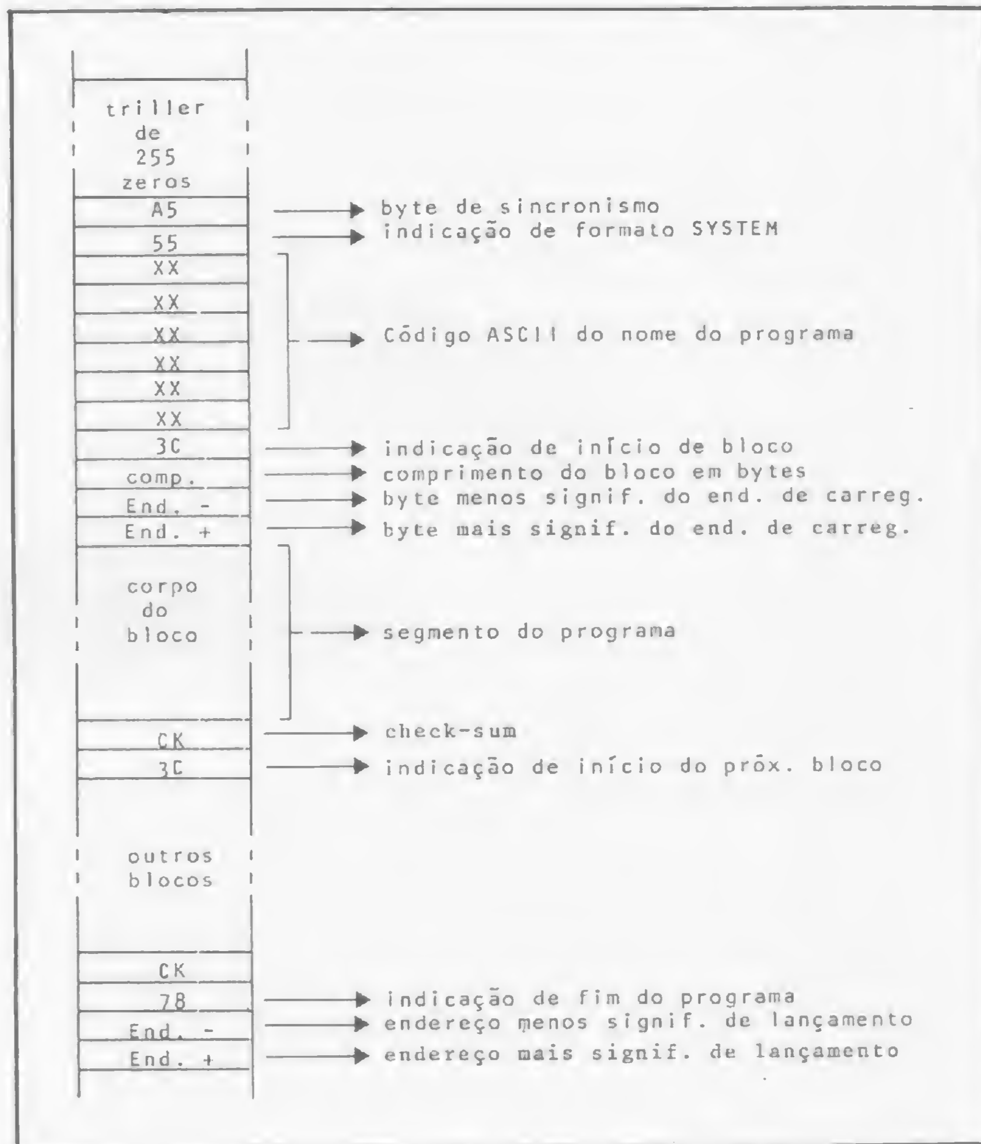
Figura 4 – Formato de uma fita SYSTEM.
